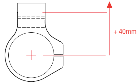
Bracciali manubrio con offset +40mm Clip-ons with +40mm offset
