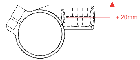
Bracciali manubrio con offset +20mm Clip-ons with +20mm offset
