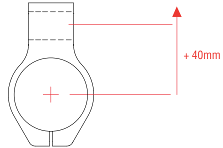
Bracciali manubrio con offset +40mm Clip-ons with +40mm offset
